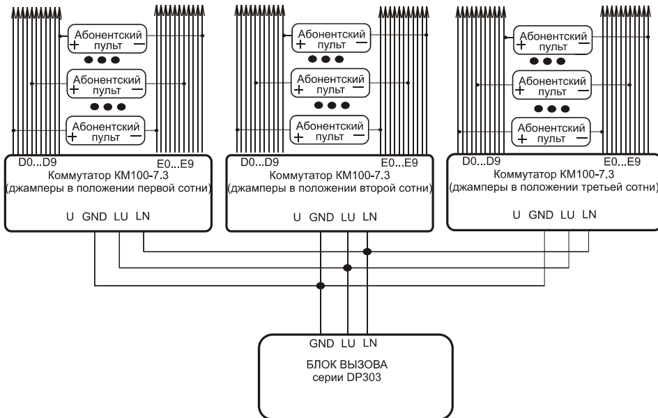
Рис.1 Вариант схемы подключения трех КМ100-7.3 на 300 абонентов
