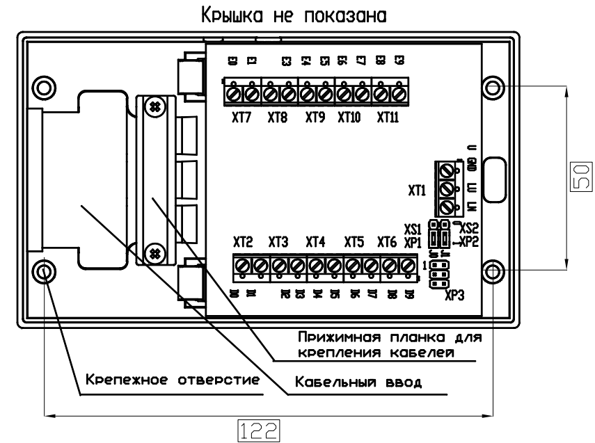
Рис. 2. Внешний вид КМ100-7.3
